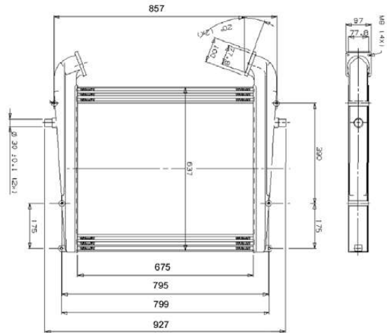
309001 675 x 637 x 62
