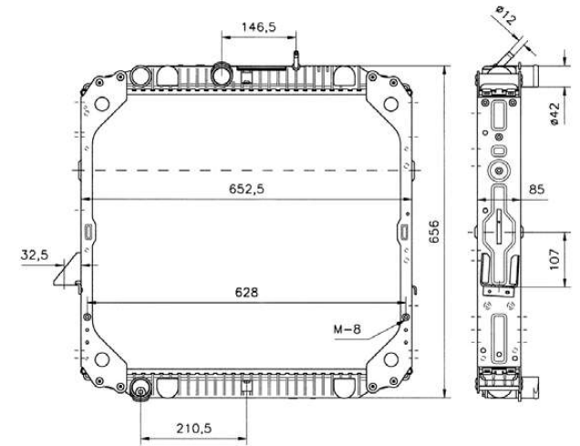
51570 544 x 618 x 43
