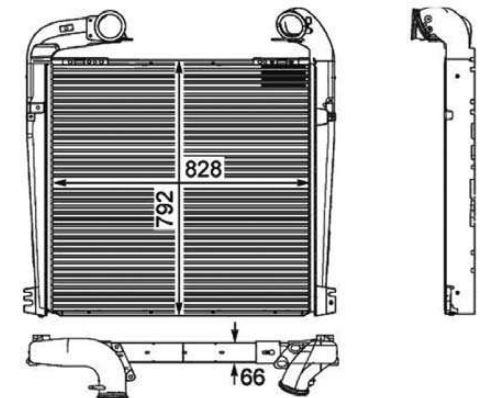
30898 792 x 828 x 66
