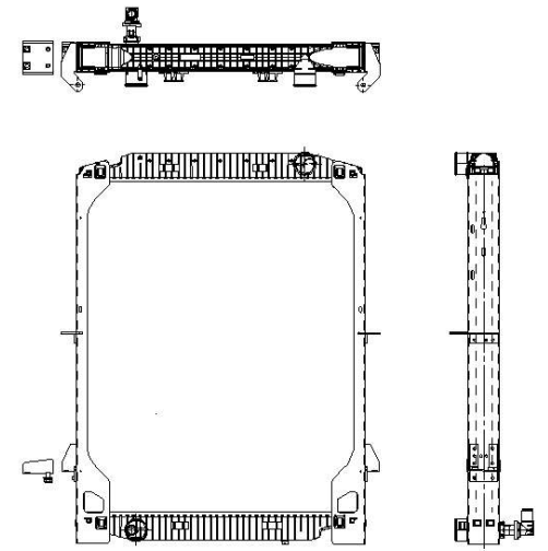
539568 900 x 773 x 43
