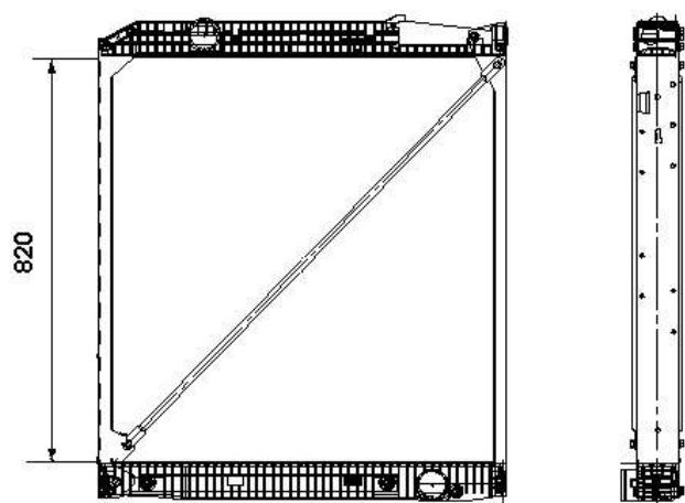
519579 820 x 829 x 48
