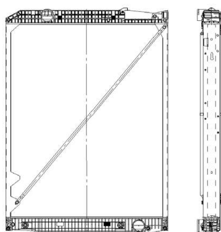
519578 1015 x 829 x 48
