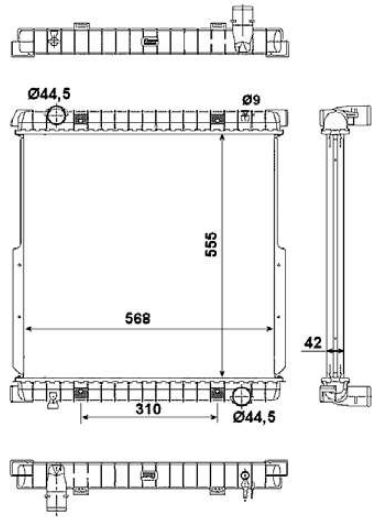
58377 555 x 568 x 42
