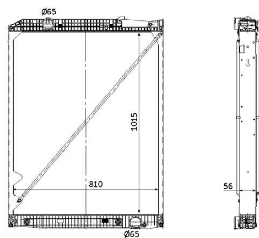
53867 1015 x 810 x 56
