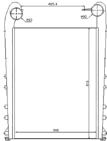
30221 593 x 815 x 65
