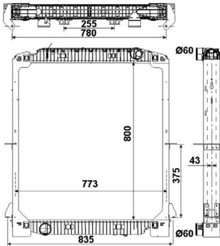
549567 800 x 773 x 43
