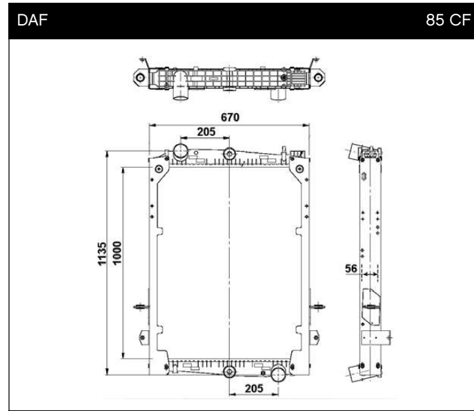
58280 1000 x 648 x 56
