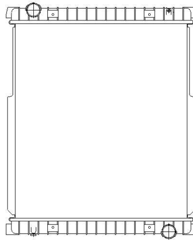
53538 640 x 565 x 42
