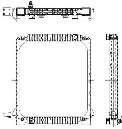
509567 800 x 773 x 43
