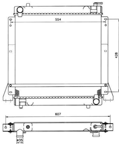
504254 480 x 501 x 34
