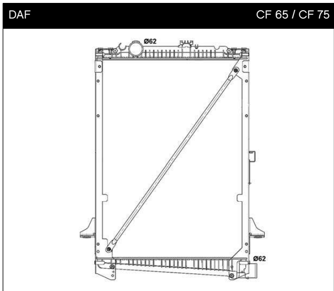
519616 850 x 648 x 56
