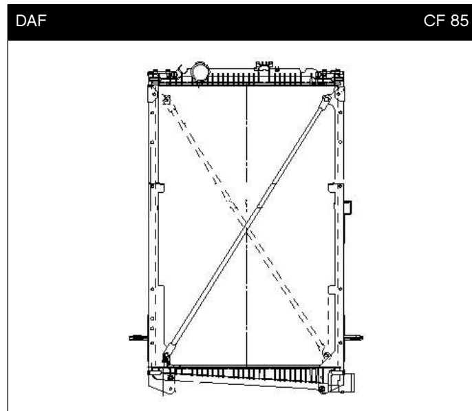
519679 950 x 648 x 56
