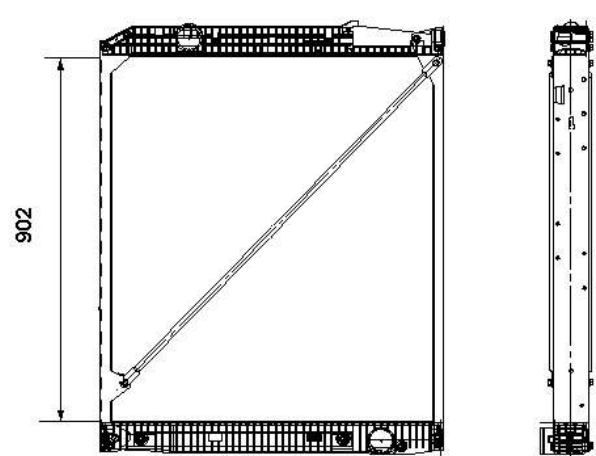
519576 902 x 829 x 48
