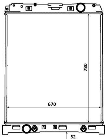
53883 780 x 670 x 52
