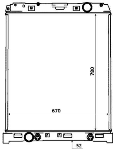
53883 780 x 670 x 52
