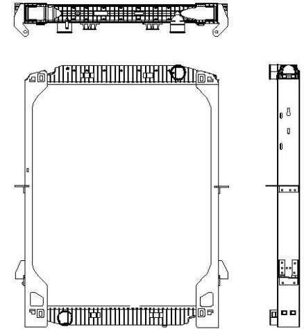
559568 900 x 773 x 43
