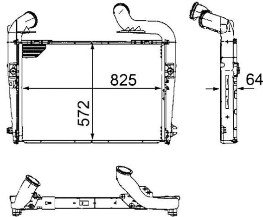
30224 825 x 572 x 64
